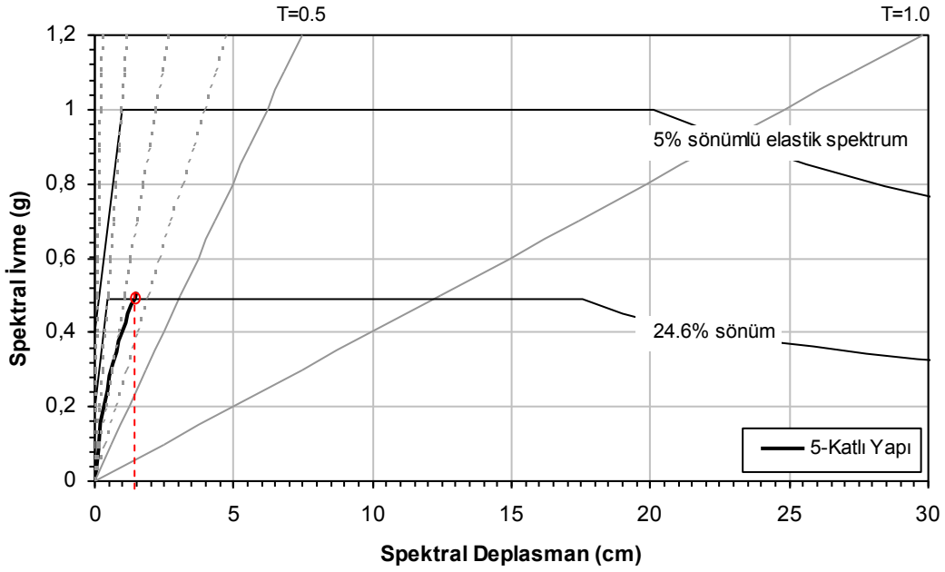
Şekil 4. Yürürlükteki deprem şartnamesi dizayn spektrumu kullanılarak 5-katlı yapı için kapasite spektrum metodunun uygulaması
